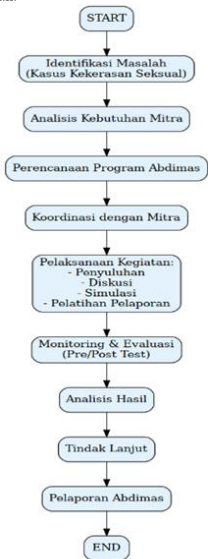
Gambar 1: Skema Metode
